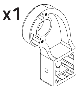
A1-A02a 147 mm
